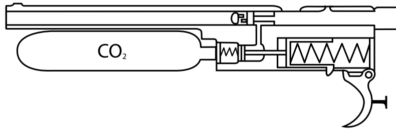
2. ábra - Sűrített gázzal működő
