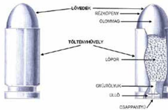
15. ábra – A lőszer részei
