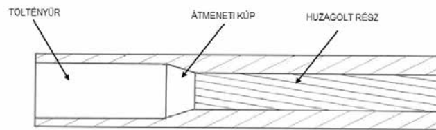
14. ábra – A fegyvercső részei
