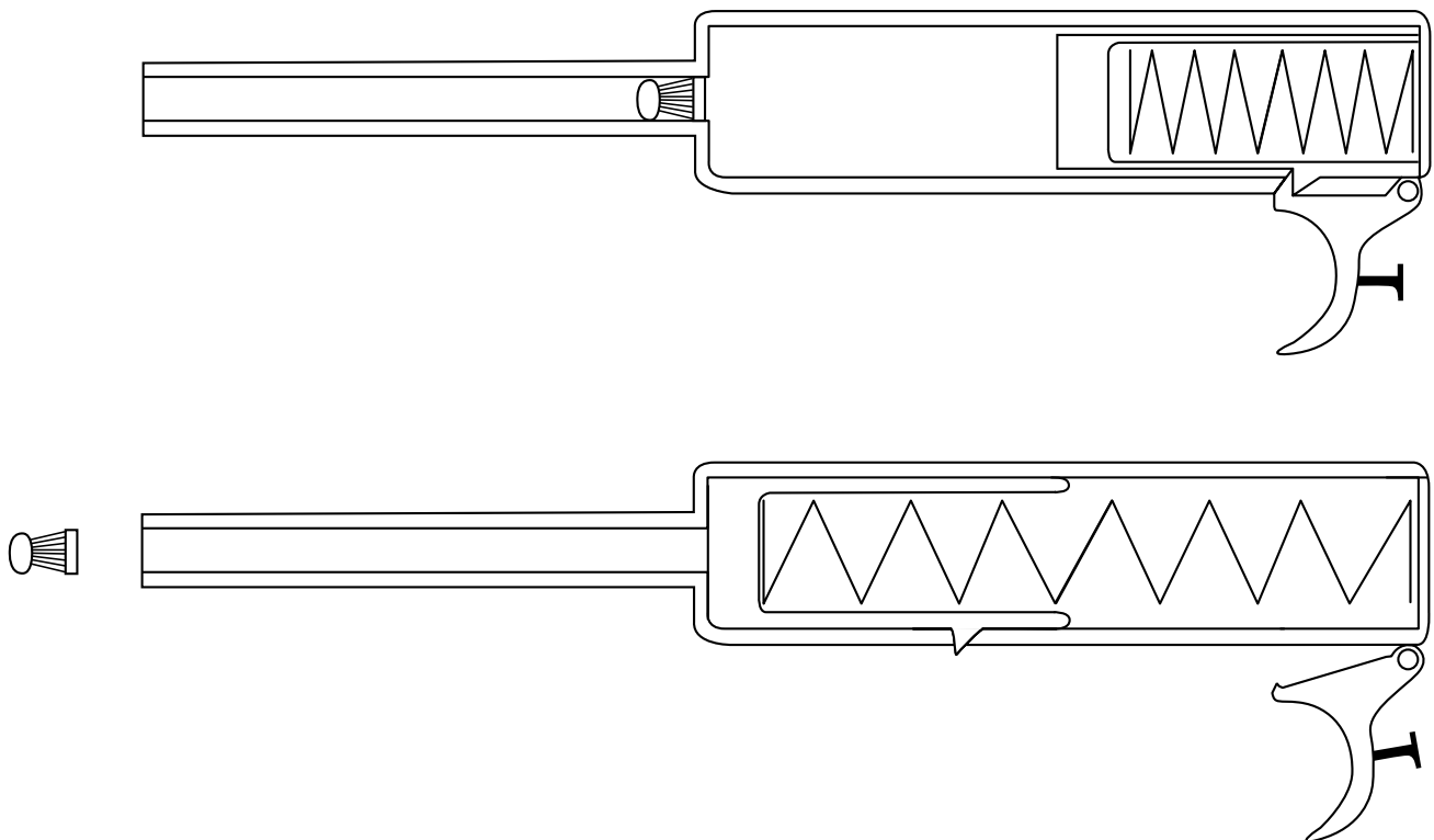
7. ábra –Lövedék előre mozgása a fegyvercsőben
