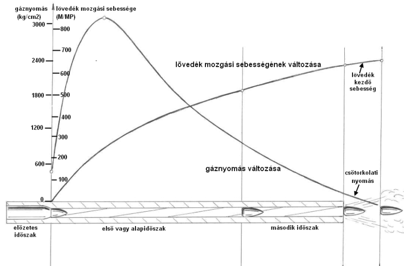
11. ábra - A lövés folyamata
