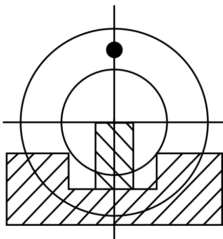
18. ábra – Durva célzás
