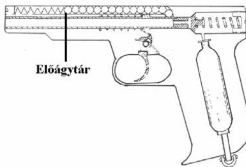
9. ábra – Ismétlő rendszerű légfegyver
