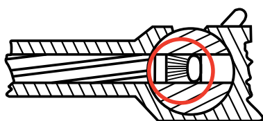
5. ábra – Zárt töltényűr
