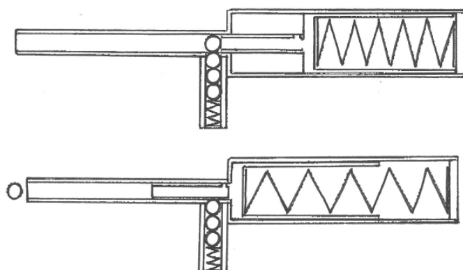
10. ábra – Lövedék kilövésének folyamata
