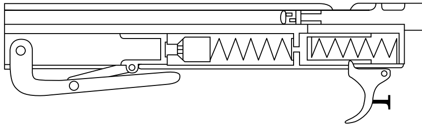
3. ábra - Pneumatikus rendszerű
