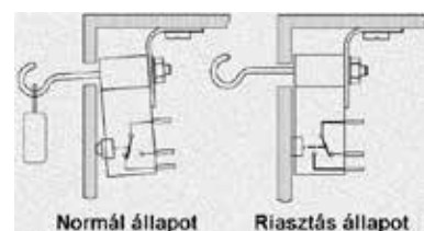
5. ábra Súlyérzékelő működés közben
